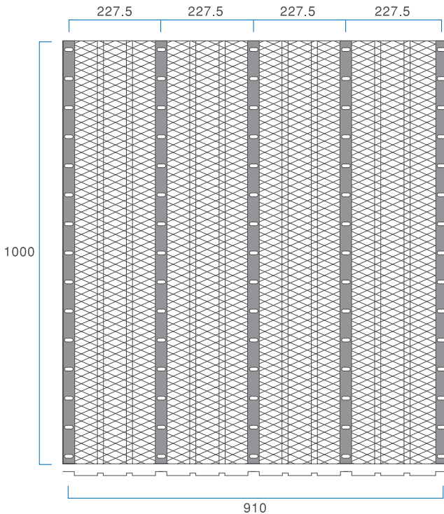
基盤形状図
